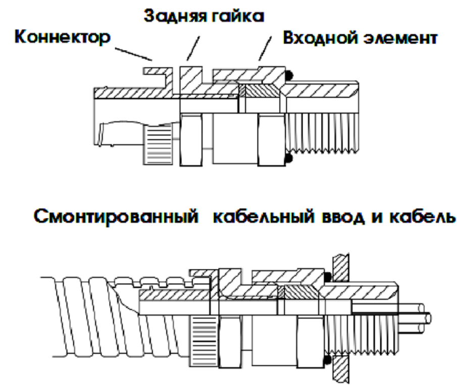
Рисунок 30 - Кабельный ввод
